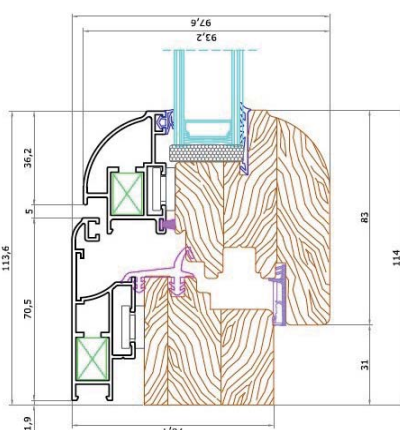
NODO VERTICALE
