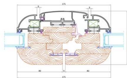
NODO CENTRALE
