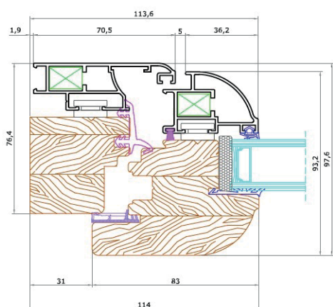
NODO ORIZZONTALE
